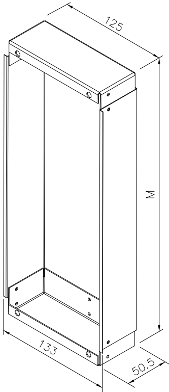
Рамка для внутреннего крепления в отверстии в стене
